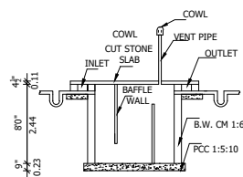
SECTION - AB
