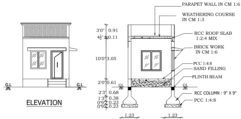
SECTION - AB
