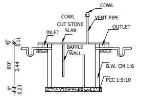
SECTION - AB
