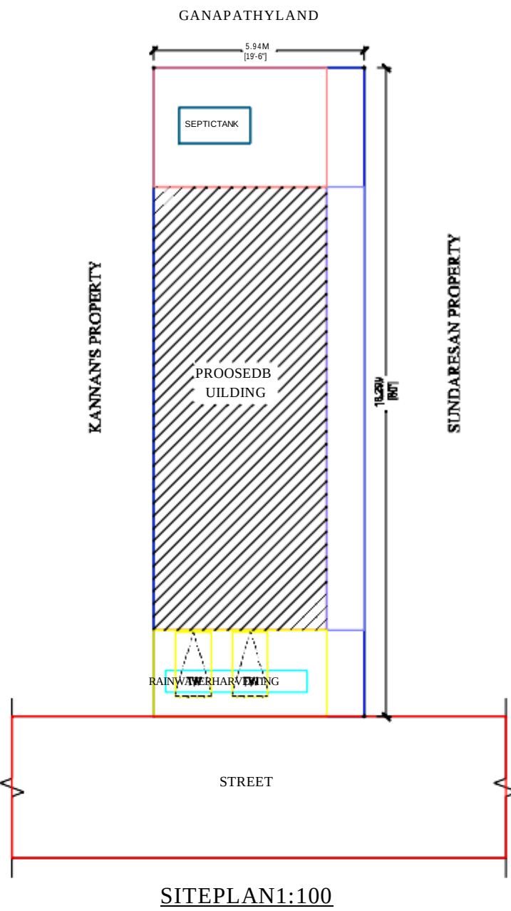
SITE PLAN 1:100
