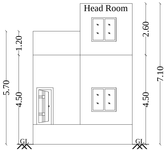
ELEVATION
