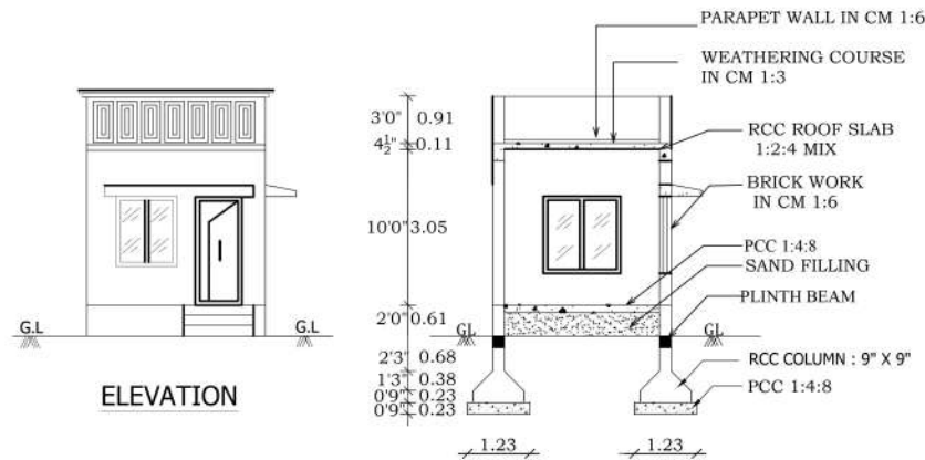
SECTION - AB
