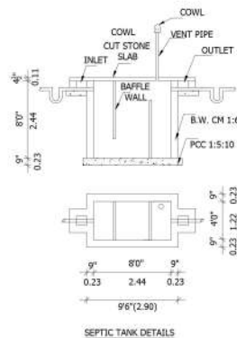
SECTION - AB
