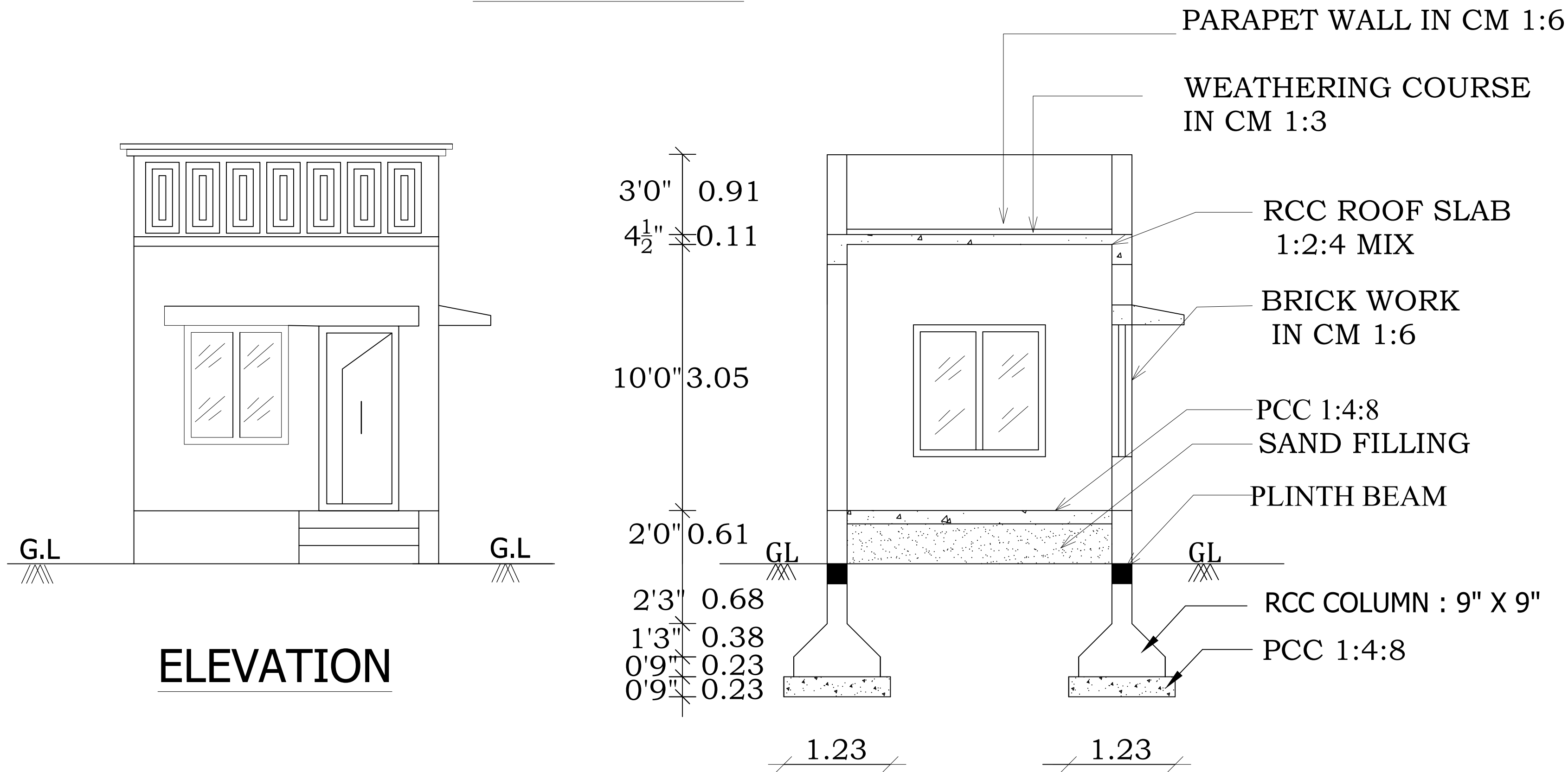
SECTION - AB
