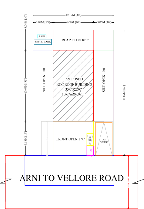
SITE PLAN(Scale 1:100)
