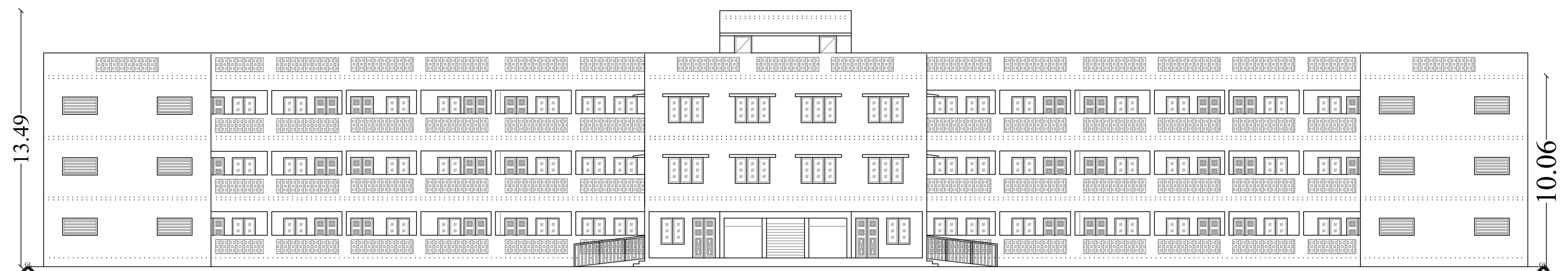
ELEVATION
