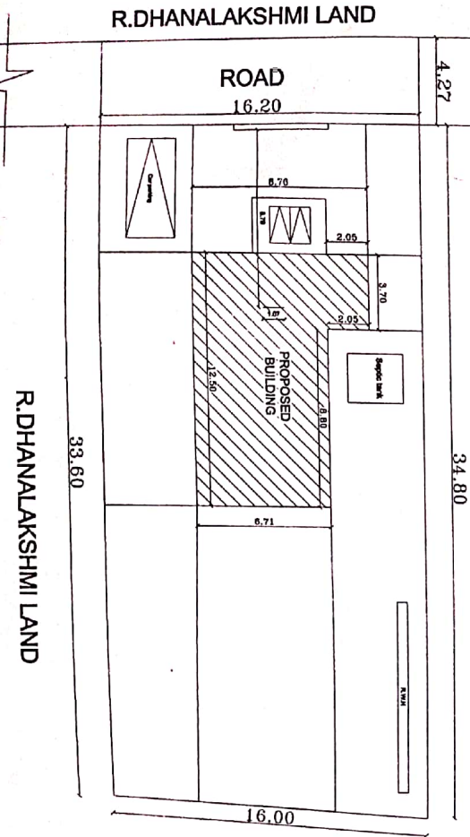
Topo Sketch SCALE:- 1:5000 MANIRETHINAM LAND
