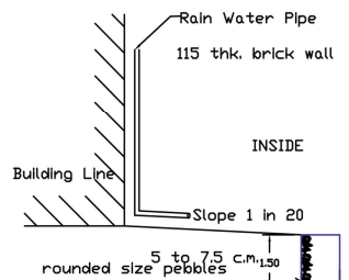
Percolation Pit.
