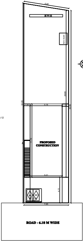
SITE PLAN - SCALE-1:100
