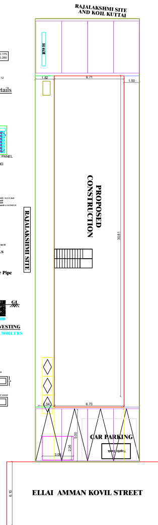
SITE PLAN - SCALE -1:100
