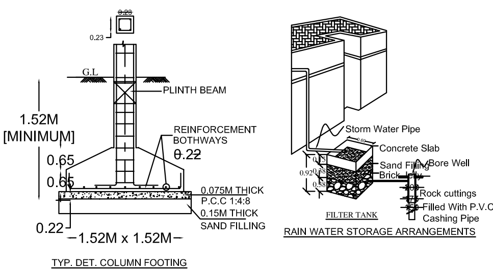
TYP. DET. COLUMN FOOTING
