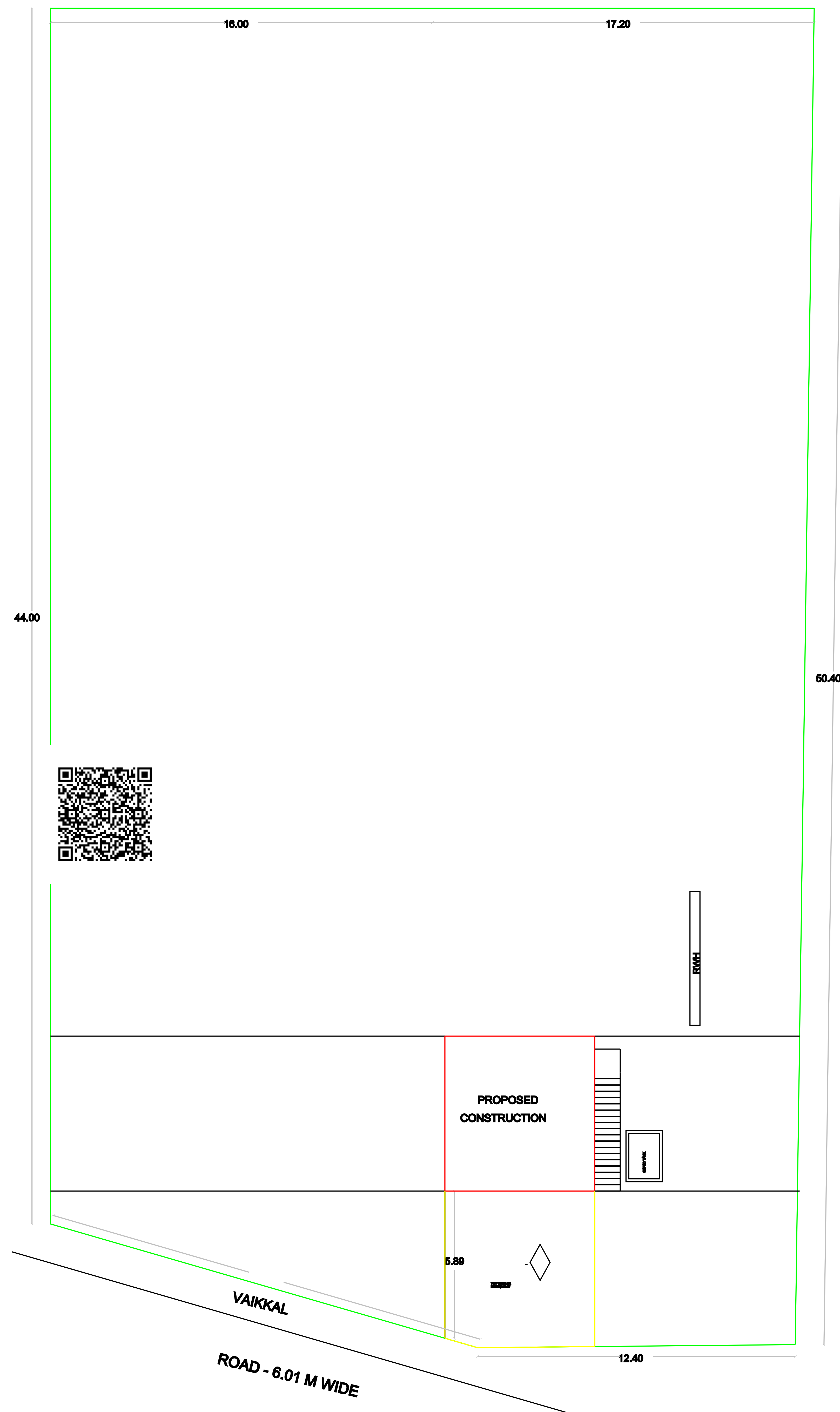
SITE PLAN SCALE - 1:100
