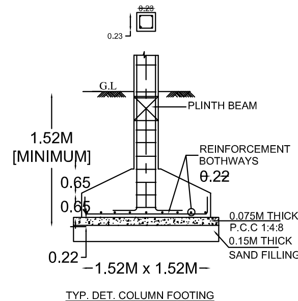
TYP. DET. COLUMN FOOTING
