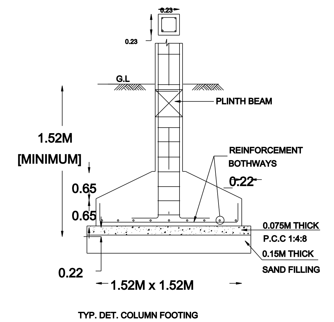
TYP. DET. COLUMN FOOTING
