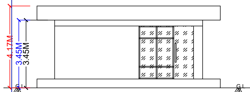
ELEVATION
