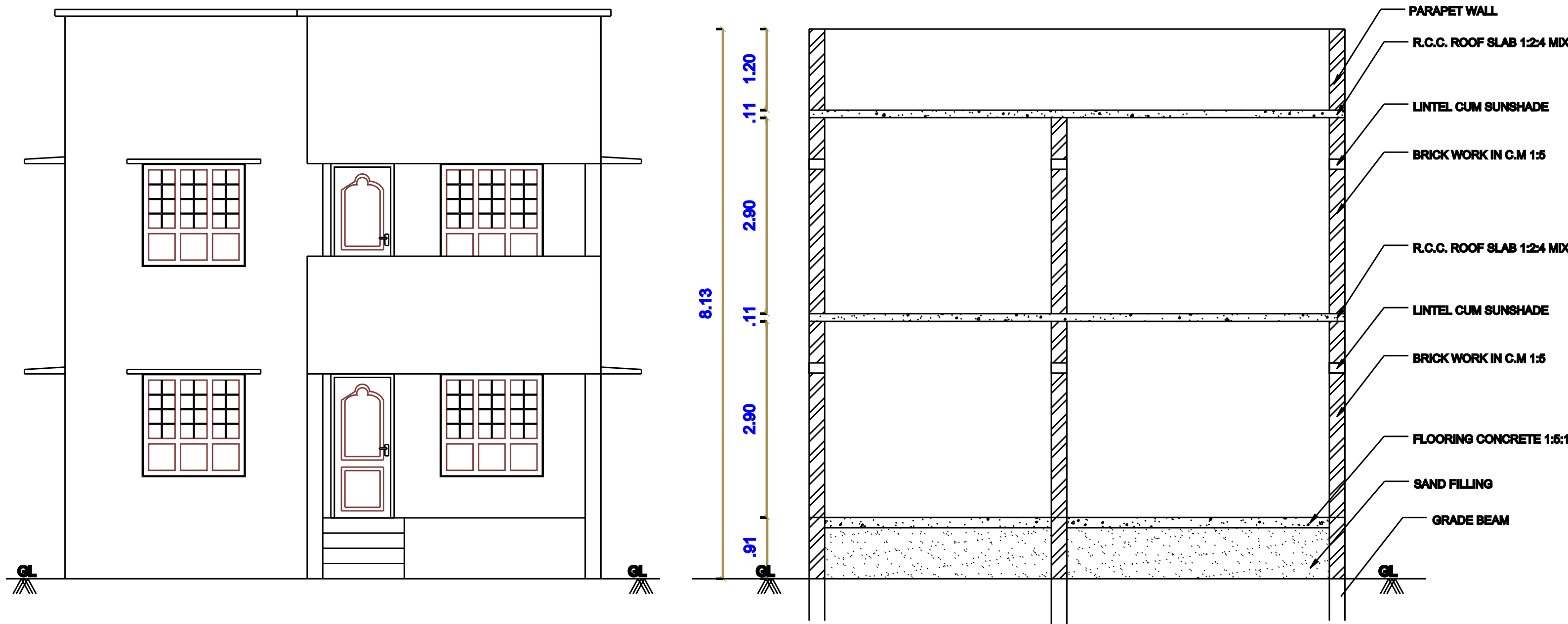
ELEVATION
