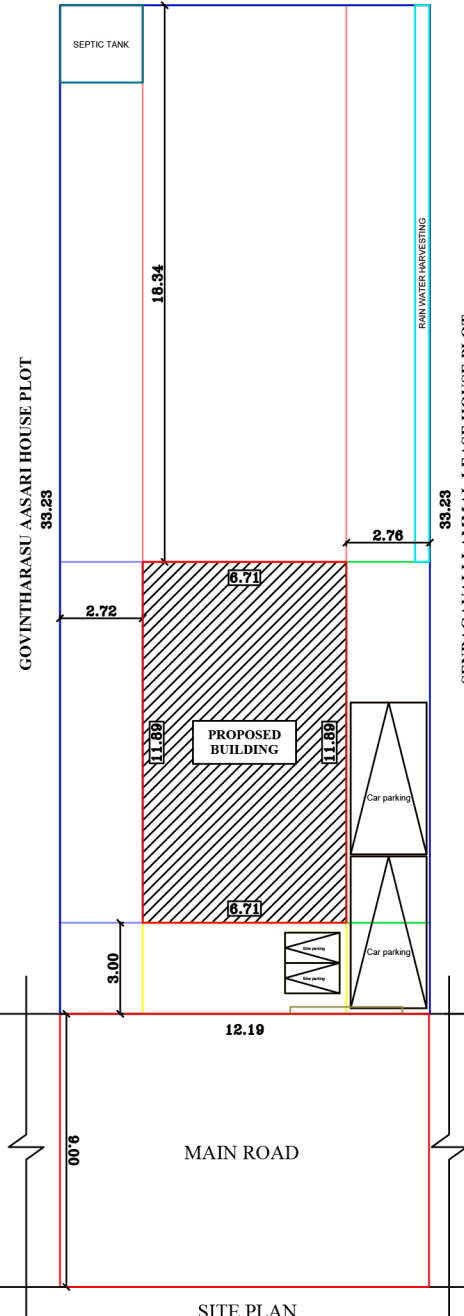
SITE PLAN SCALE 1:100
