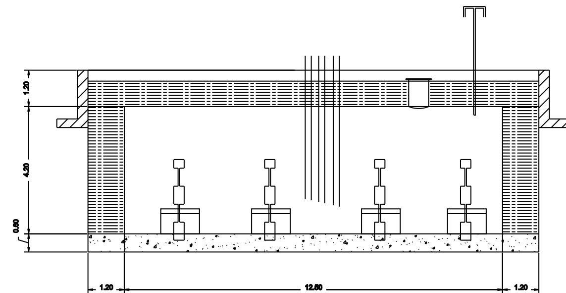
LONGITUDINAL SECTION
