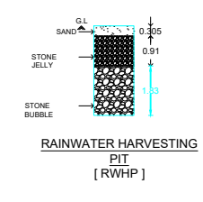
RAINWATER HARVESTING [R.W.H.P.]
