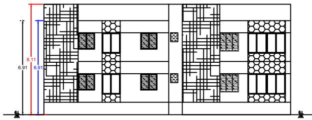
ELEVATION
