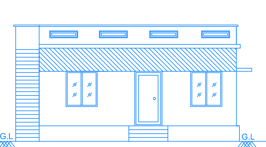
ELEVATION
