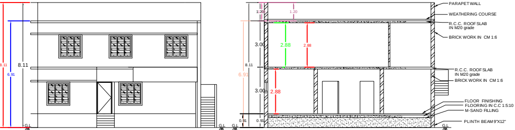
ELEVATION
