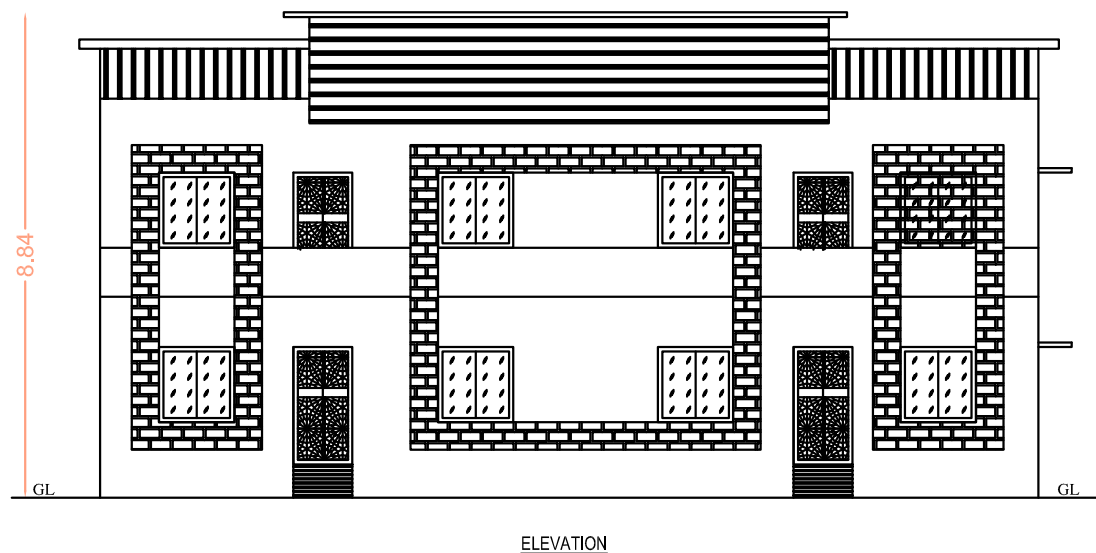
ELEVATION
