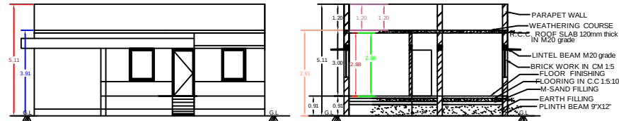
ELEVATION
