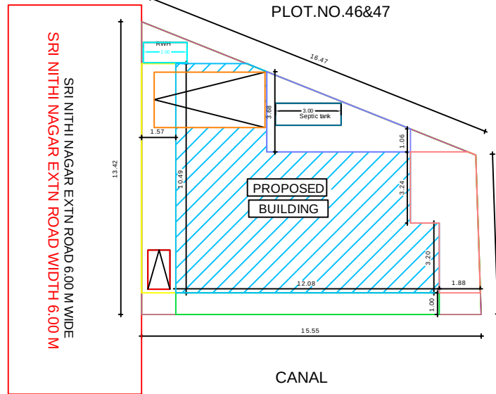
PLOT.NO.46&47
