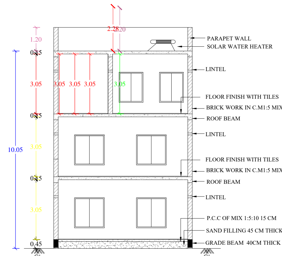
SECTION -AB
