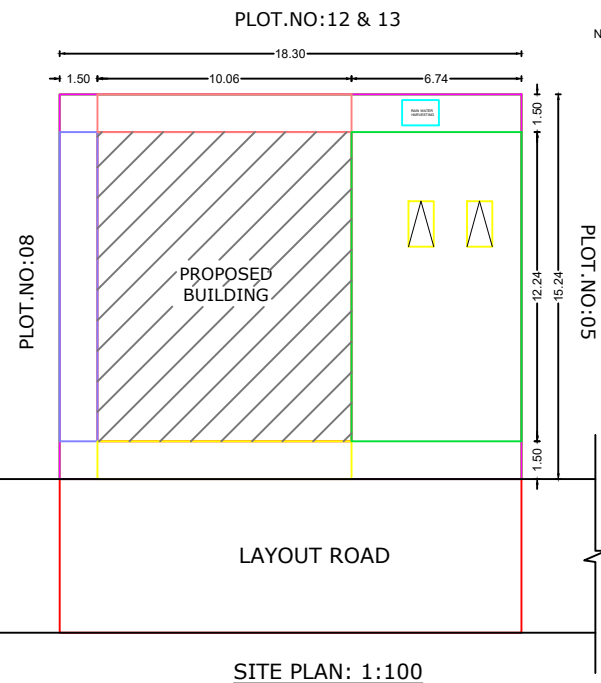
SITE PLAN: 1:100
