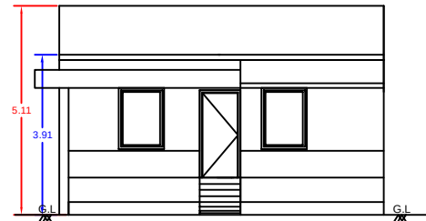
ELEVATION
