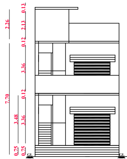
ELEVATION B-B'
