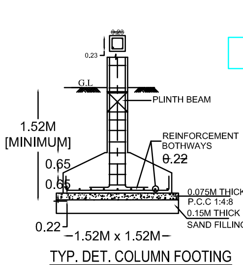
TYP. DET. COLUMN FOOTING
