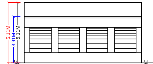
ELEVATION
