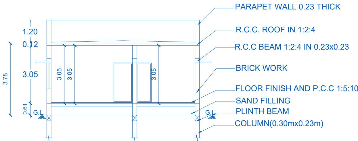
SECTION A-B
