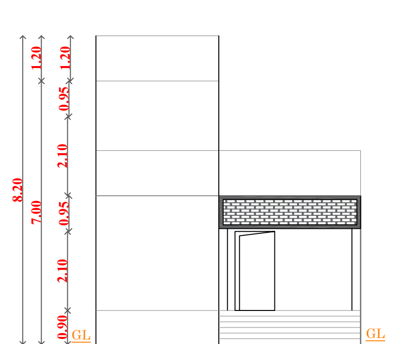
ELEVATION B-B'
