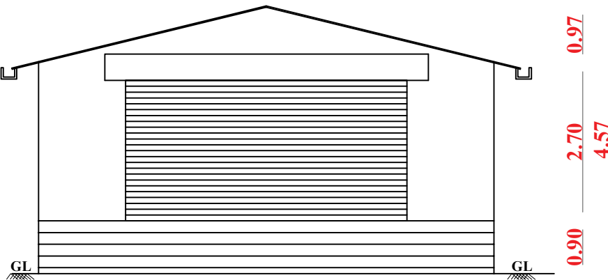
ELEVATION B-B'
