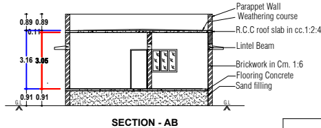
SECTION - AB
