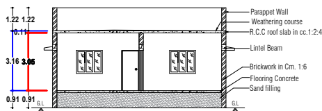
SECTION - AB
