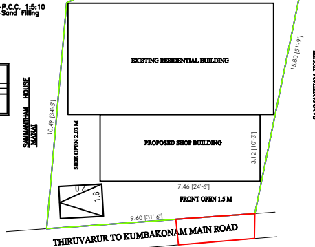
SITE PLAN SCALE 1:100
