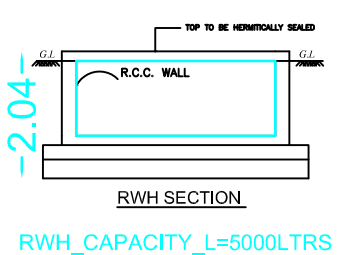
RW H_CAPACITY_L=5000LTRS
