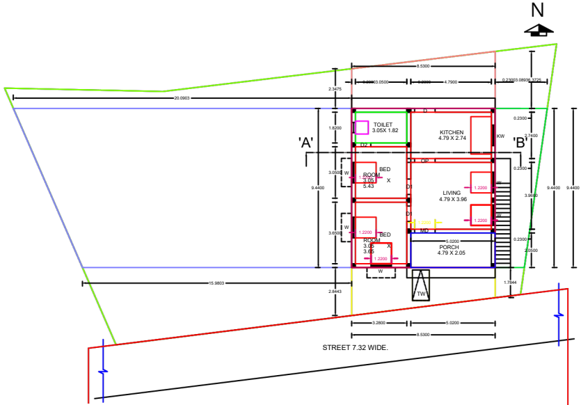
UND FLOOR PLAN.
