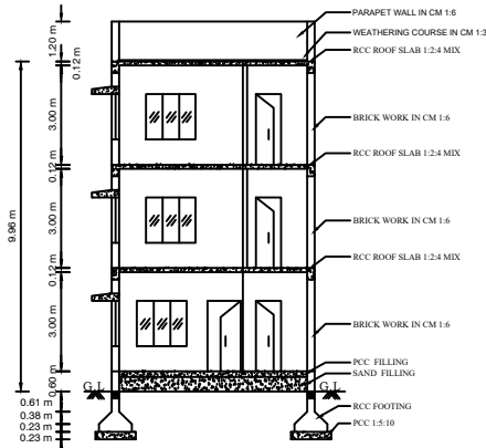
SECTION - AB
