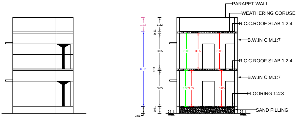
ELEVATION
