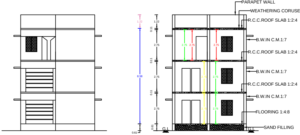
ELEVATION
