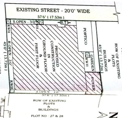
SITE PLAN SCALE: 1:200
