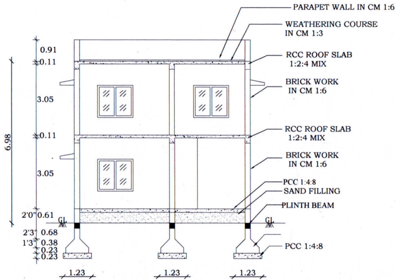
SECTION - AB
