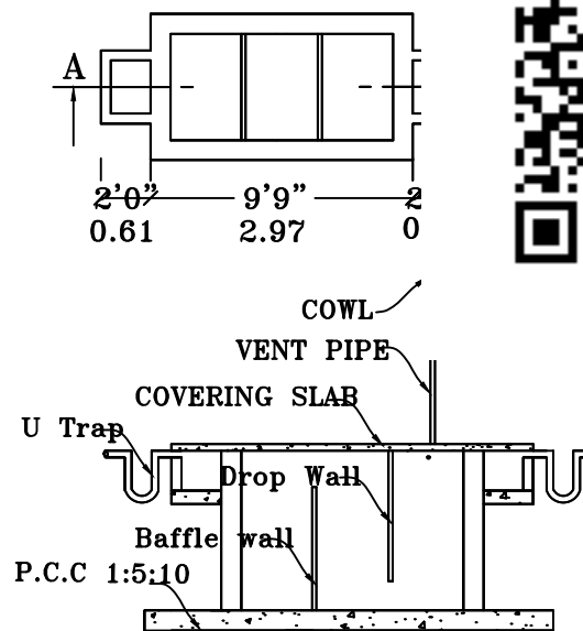
SEPTIC TANK DE
