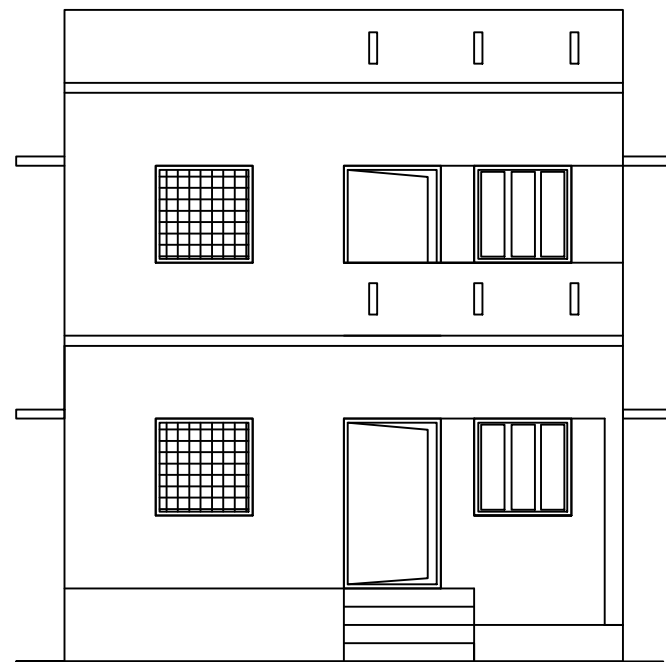
ELEVATION
