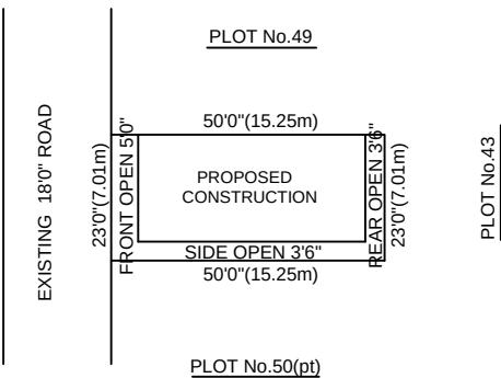
SITE PLAN:
