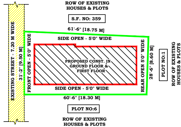
SITE PLAN:
