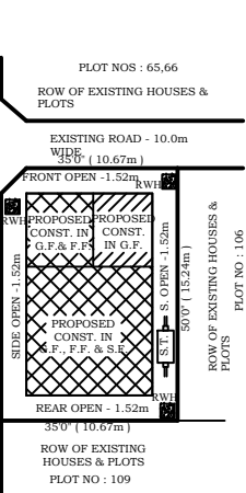
SITE PLAN SCALE : 1:200
